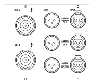
Fig. 29: D12 Anschlussplatte NL8
