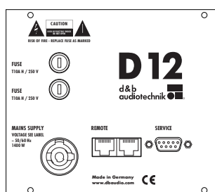
Fig. 26: D12 Netzurückplatte
